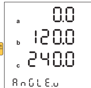
Phase voltage phase angle V1-V1 V2-V1 V3-V1
