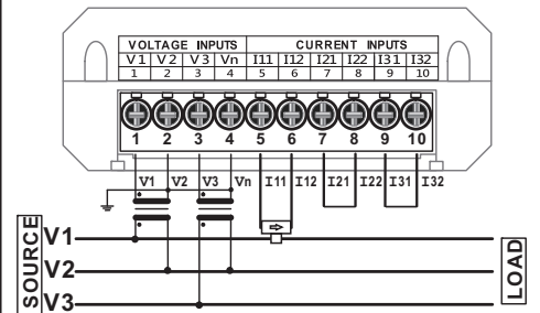
1CT(0~333mV)
