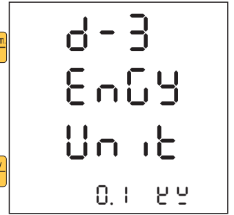
Energy unit 0.0001kWh / 0.001kWh 0.01kWh / 0.1kWh / 1kWh / 0.01MWh / 0.1MWh
