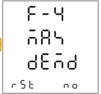
Reset Maximum demand: NO/YES
